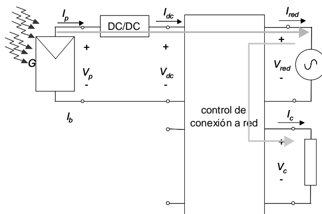
Fig. 1: Diagrama de bloques del Sistema.
