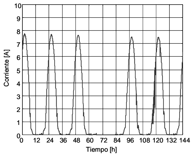
Fig. 4: Corriente a la salida del generador fotovoltaico.
