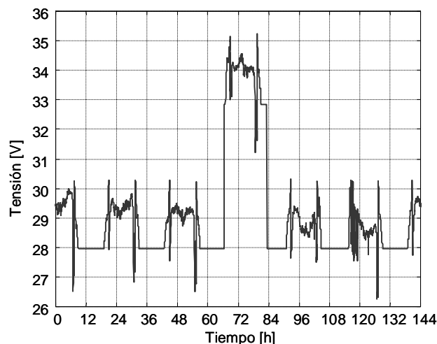
Fig. 3: Evolución de la tensión de salida del generador fotovoltaico.
